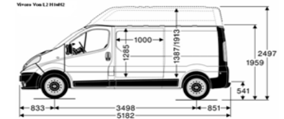
Vivaro Van L2 H1482
