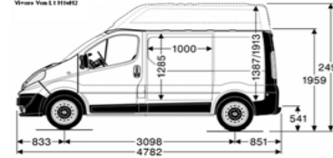
Vivaro Van L1 H1482
